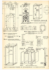
Mechanischer Zusammenbau
