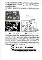
CTR Miniatursender KM 2/5
