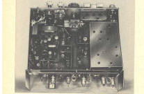
Bild 92. Innensicht der 2-m-Station von DL 9 IW.
