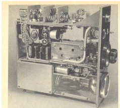
Bild 87. 2-m-Station von DL 9 AL. Innensicht von der Tuner-Seite.
