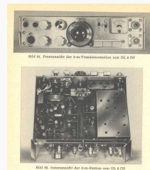
Transistorstation von DL9AL
