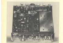
Bild 91. Innensicht der 2-m-Station von DL 9 AL
