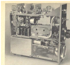
Bild 89. 2-m-Station von DL9AL. Innensicht von der Tuner-Seite
