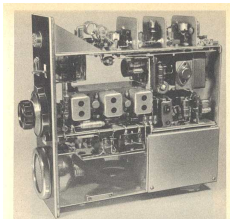
Bild 88. Innenansicht der 2-m-Station von DL 9 AL mit Zf-Baustein
