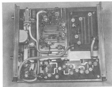
Bild 92. Innenaussicht des 70cm-Zustückgerätes von DL 6 MH.
