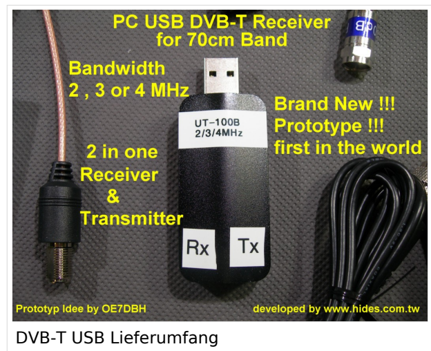
DVB-T USB Prototyp
