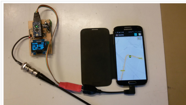
LoRa Empfänger mit angeschlossenem Handy mit Positionsanzeige via W2APRS
